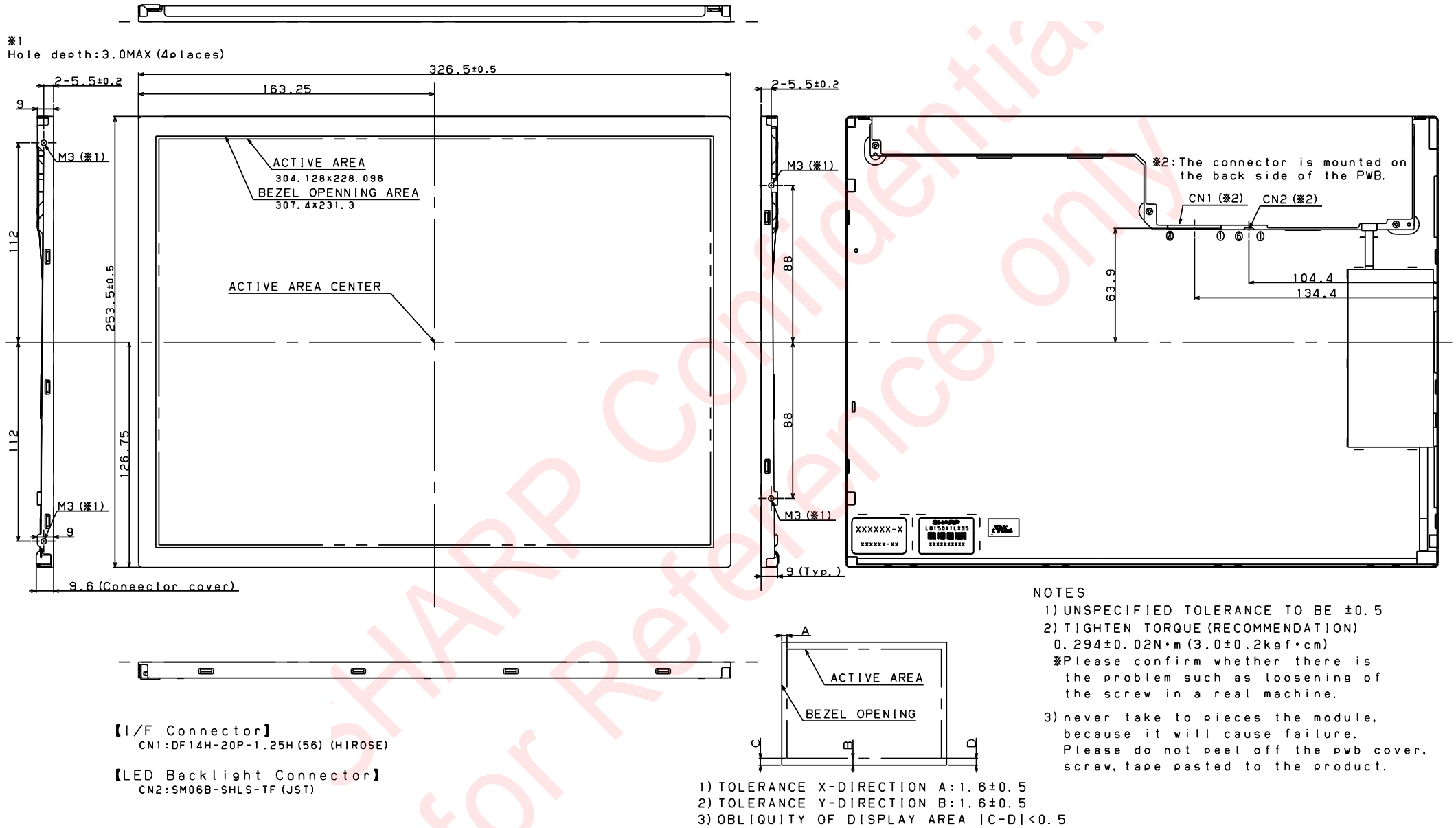
图1. LQ150X1LX95外形寸法图 Fig.1. Outline Dimensions
