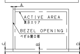
Bezel/Display position ベゼル/画面位置詳細
